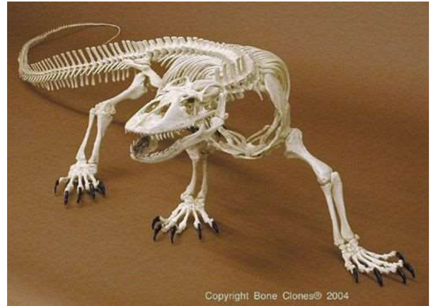
Komodo Dragon
