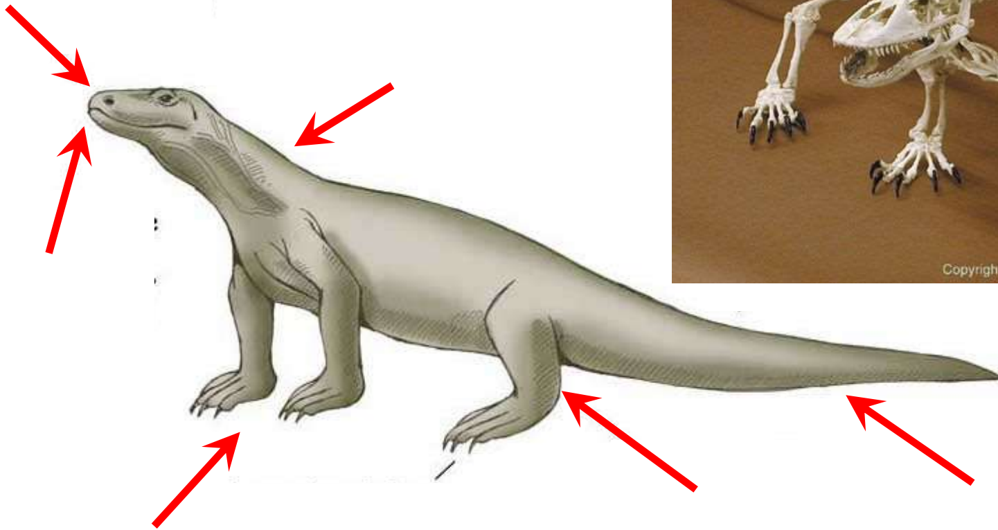
Komodo Dragon
